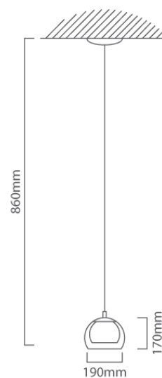
P208 CAD DIAGRAM
