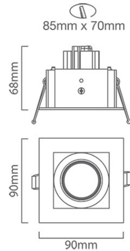
PR345 CAD DIAGRAM
