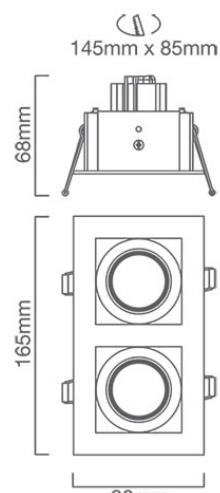
PR346 CAD DIAGRAM
