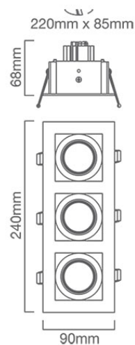
PR347 CAD DIAGRAM
